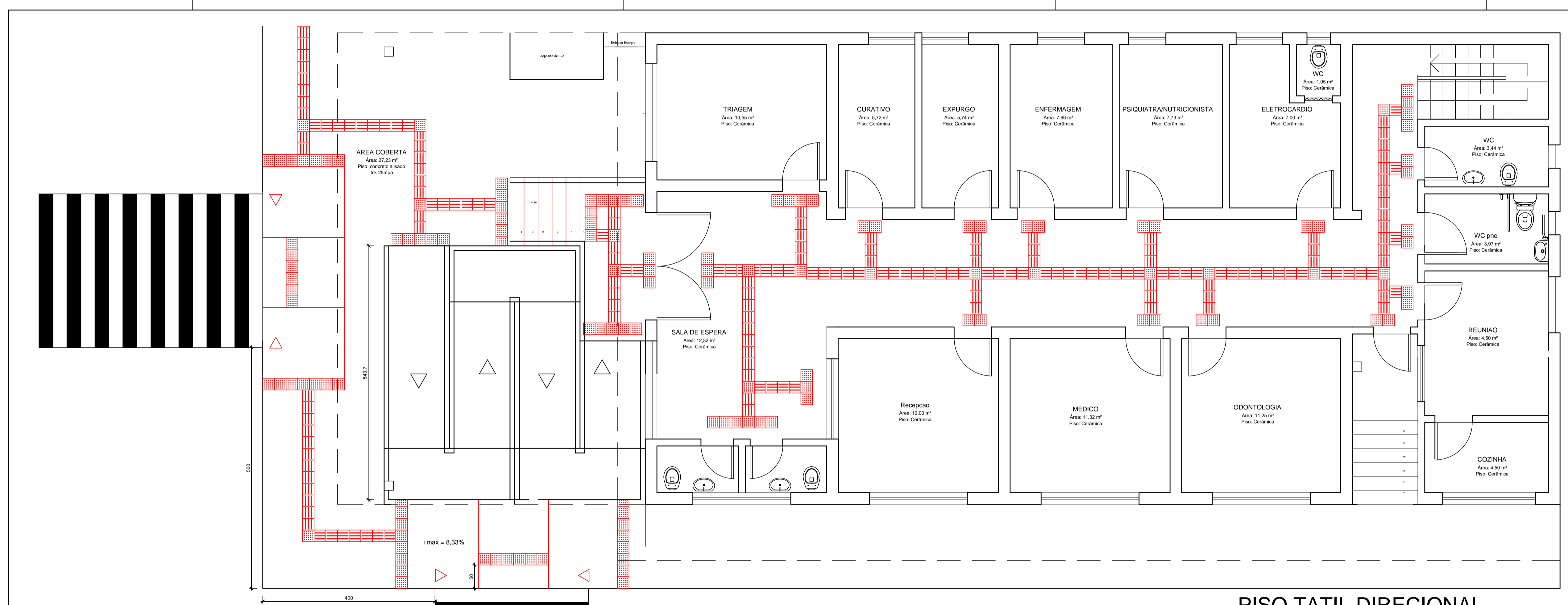
PISO TATIL DIRECIONAL ESCALA: 1:50
