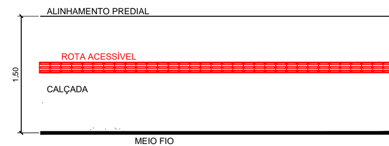
DETALHE DO PASSEIO SEM ESCALA
