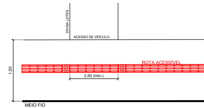
DETALHE ACESSO DE VEÍCULO SEM ESCALA
