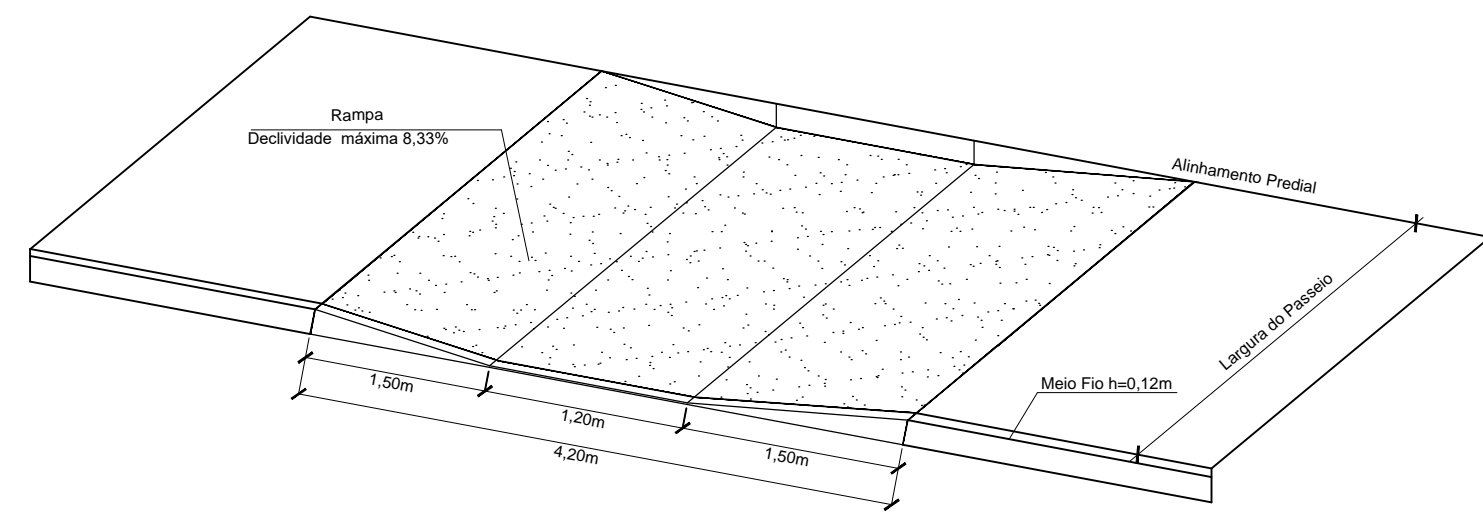
DETALHE RAMPA DE ACESSO SEM ESCALA
