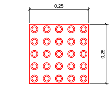
DETALHE PISO TÁTIL DE ALERTA SEM ESCALA
