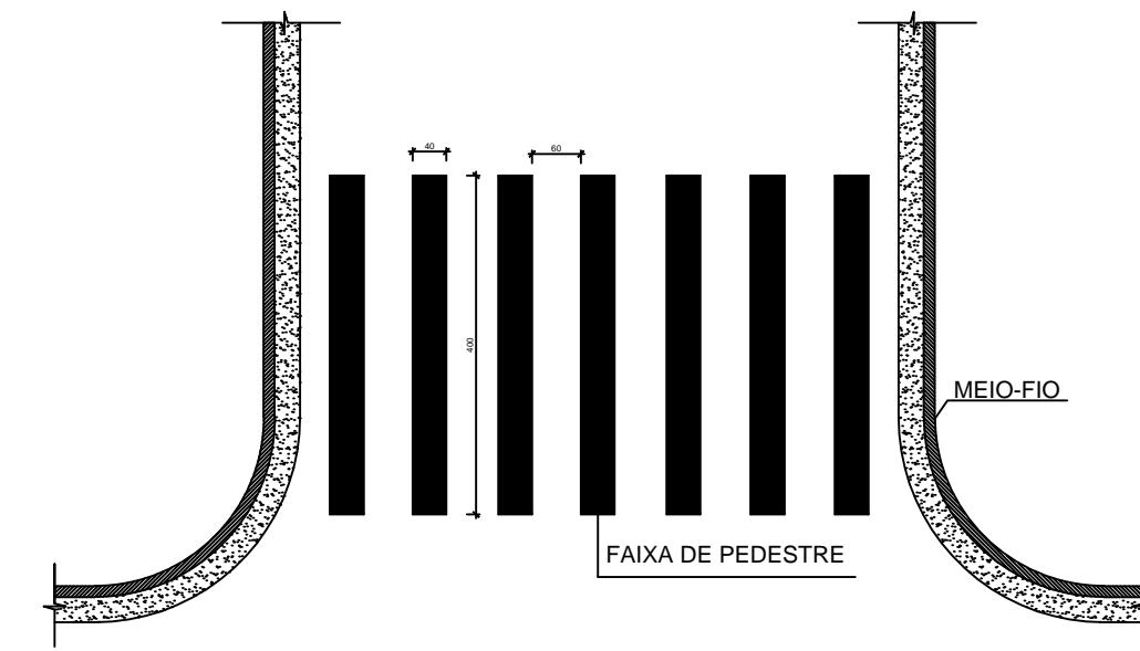
ACESSIBILIDADE - REBAIXO DE MEIO-FIO E DETALHE DE FAIXA DE PEDESTRE ZEBRADA Tinta: EXTRUDADO Cor: BRANCA
