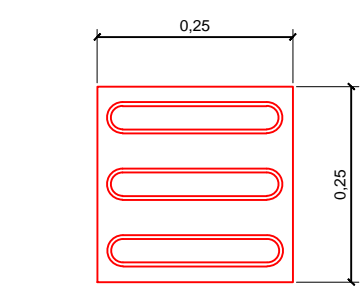
DETALHE PISO TÁTIL DIRECIONAL SEM ESCALA
