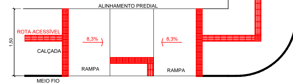
DETALHE DAS ESQUINAS SEM ESCALA
